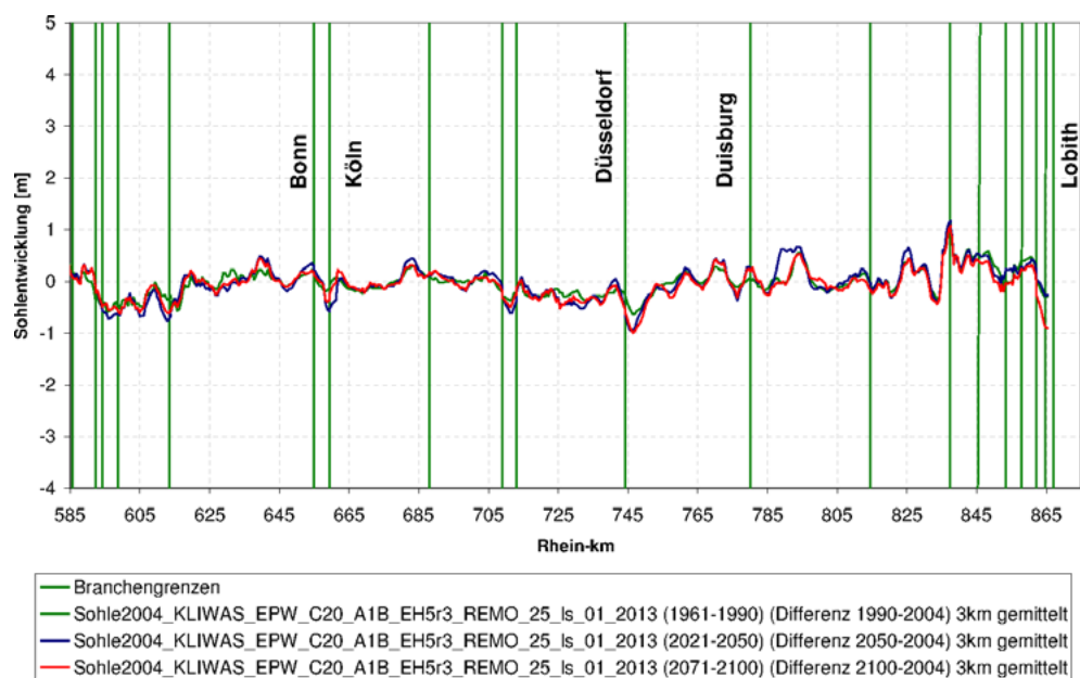
Abbildung 13: Relative Sohlentwicklung am Niederrhein für den Referenzzeitraum, die nahe Zukunft und die ferne Zukunft für die Projektion HBV134-EPW-C20_A1B_EH5r3_Remo_25_Is bezogen jeweils auf das Jahr 2004
