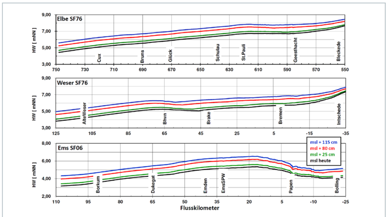
Abbildung 6: Sturmflutscheitelwasserstand entlang der Ästuar von Elbe, Weser und Ems bei heutigem Meeresspiegel (schwarz) sowie bei einem Meeresspiegelanstieg von +25 cm (grün), +80 cm (rot) oder +115 cm (blau)
