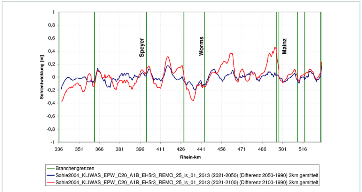
Abbildung 14: Relative Sohlentwicklung am Oberrhein in der nahen und fernen Zukunft für die Projektion HBV134-EPW-C20_A1B_EH5r3_Remo_25_Is bezogen auf den Referenzzeitraum 1961 bis 1990 (Null-Linie)
