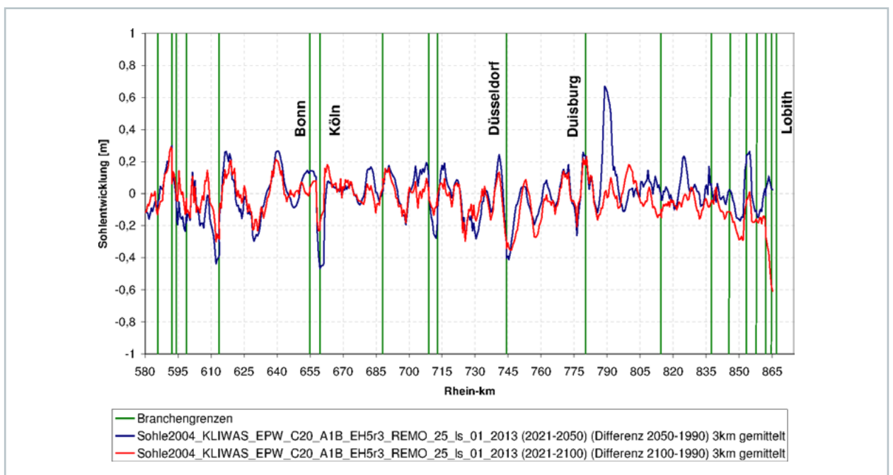
Abbildung 15: Relative Sohlentwicklung am Niederrhein in der nahen und fernen Zukunft für die Projektionen HBV134-EPW-C20_A1B_EH5r3_Remo_25_Is bezogen auf den Referenzzeitraum 1961 bis 1990 (Null-Linie)
