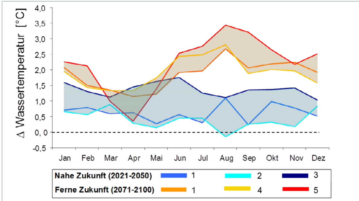
Abbildung 16: Projizierte Änderungen der Wassertemperatur (Bandbreite der Monatsmittel) in der nahen (blau) und fernen (rot) Zukunft verglichen mit der Referenzperiode (1961 bis 1990). Dargestellt sind Mittelwerte von neun Messstationen auf der frei fließenden Rheinstrecke zwischen Karlsruhe und Bimmen
