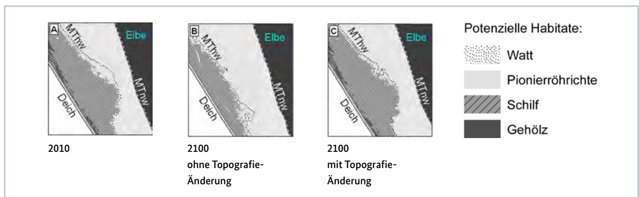
Abbildung 11: Habitatänderung an der Elbe (Wischhafen), basierend auf zwei Szenarien. A: Referenzdaten 2010, B und C: Modellerte Vegetationsverteilung 2100 ohne / mit Topografieänderung (=Mitwachsen der Vorlandflächen durch Sedimentation) (Abbildung aus Fuchs et. al. 2013)
