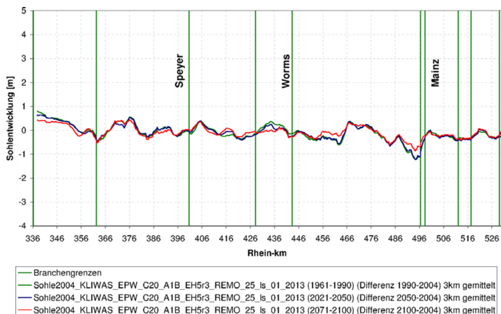
Abbildung 12: Relative Sohlentwicklung am Oberrhein für den Referenzzeitraum, die nahe Zukunft und die ferne Zukunft für die Projektion HBV134-EPW-C20_A1B_EH5r3_Remo_25_Is bezogen jeweils auf das Jahr 2004 (Null-Linie)
