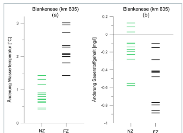
Abbildung 10: Änderung des Saisonmittelwertes (01.04. – 31.10.) a) der Wassertemperatur und b) des Sauerstoffgehalts im Elbe-Ästuar an der Station Blankenese (km 635) für die nahe Zukunft (NZ) und die ferne Zukunft (FZ)
